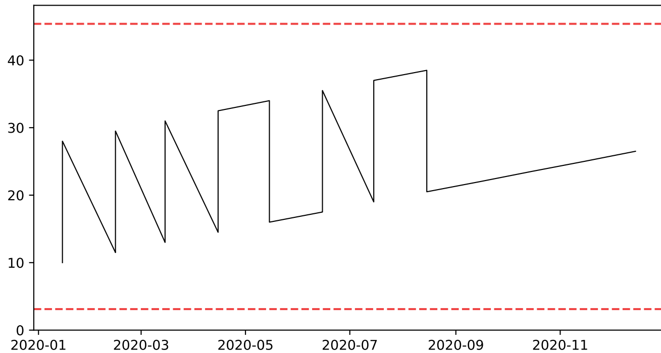
Datos Atípicos
